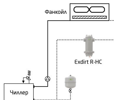
Exdirt R-NC - пример монтажа
