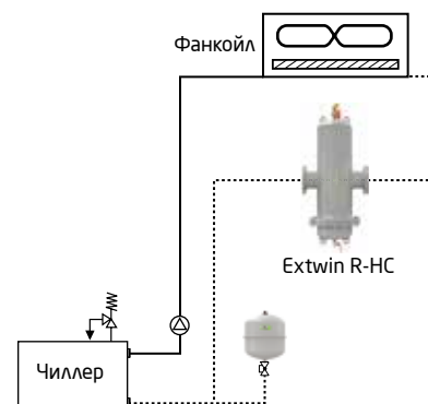
Extwin R-HC - пример монтажа
