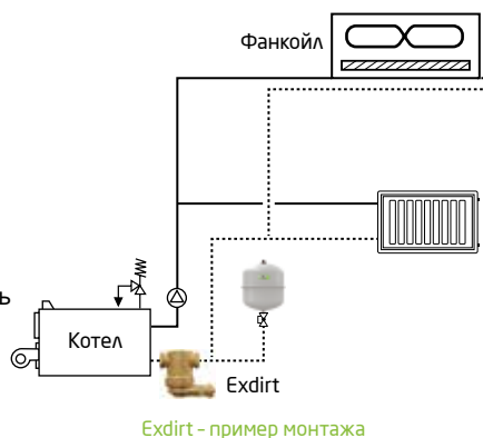
Exdirt - пример монтажа
